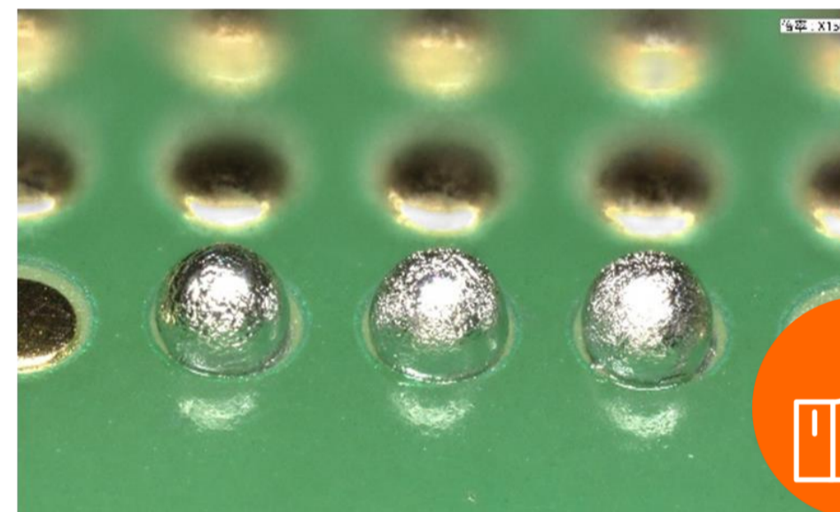
錫球保持獨立並熔融於基板
