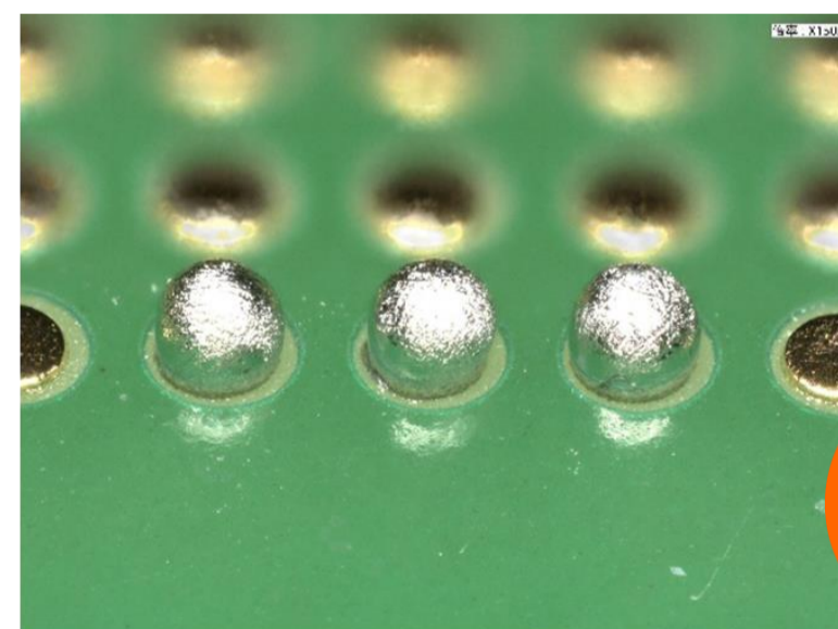
錫球表面平順
