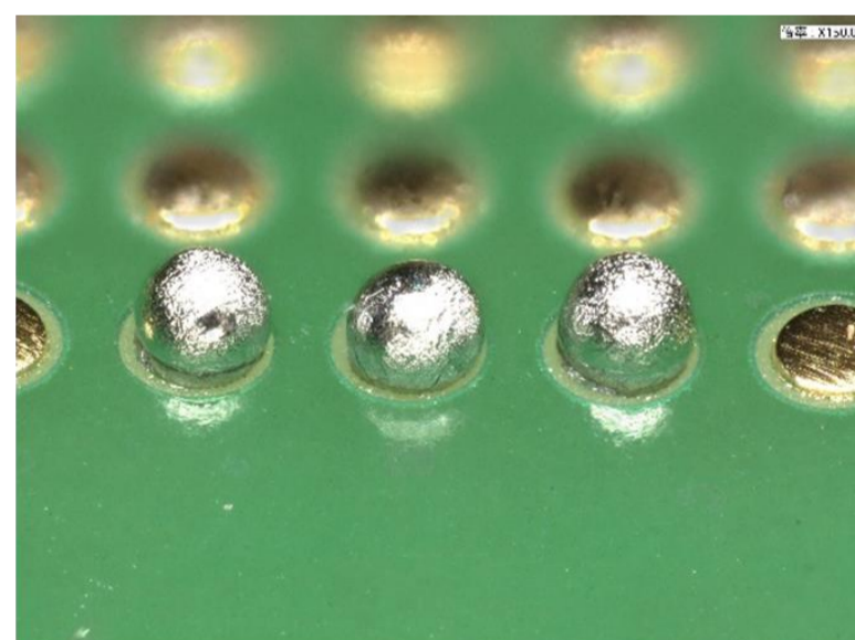
錫球表面凹陷
