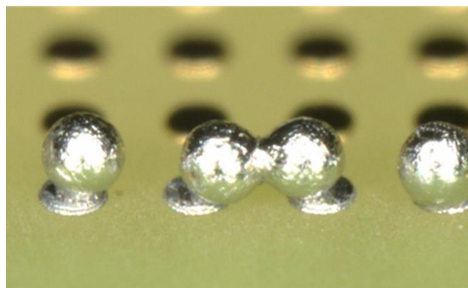
相鄰的錫球連接
